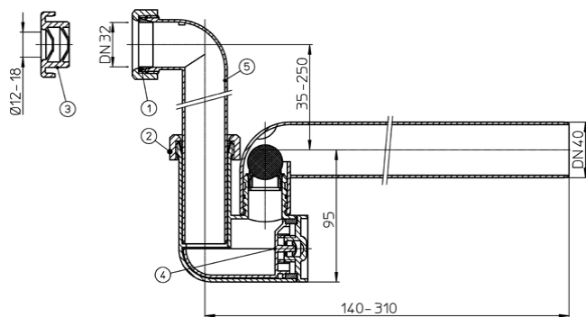
Рис. 1. Сифон HL136N.
